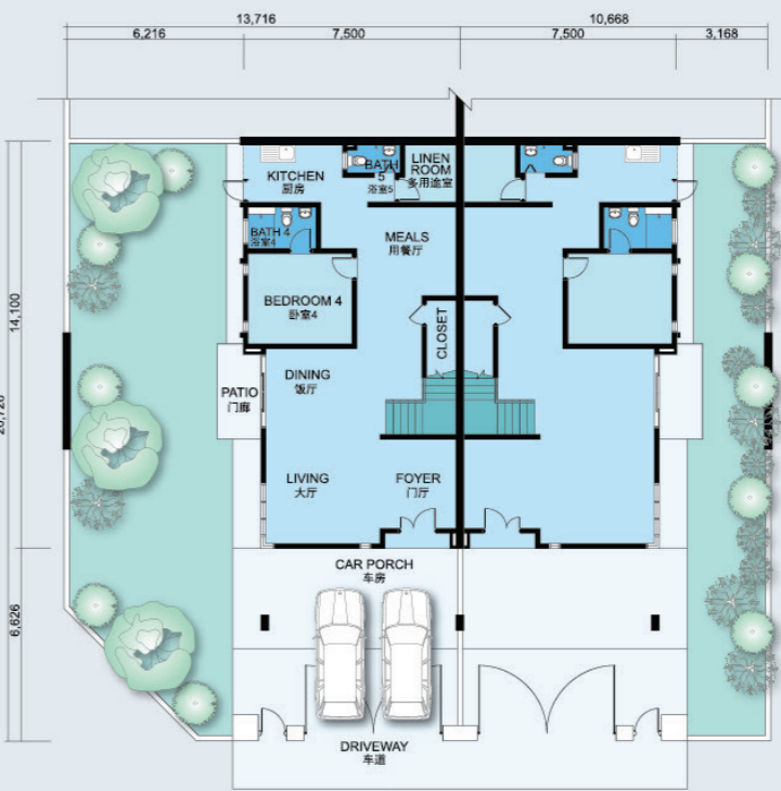
Ground Floor 底楼平面图
